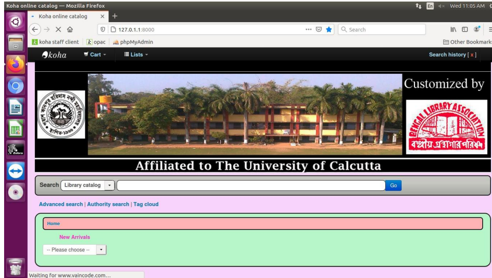
KOHA Interface
